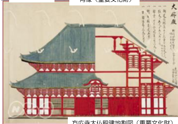
方広寺大仏殿建地割図 (重要文化財)
